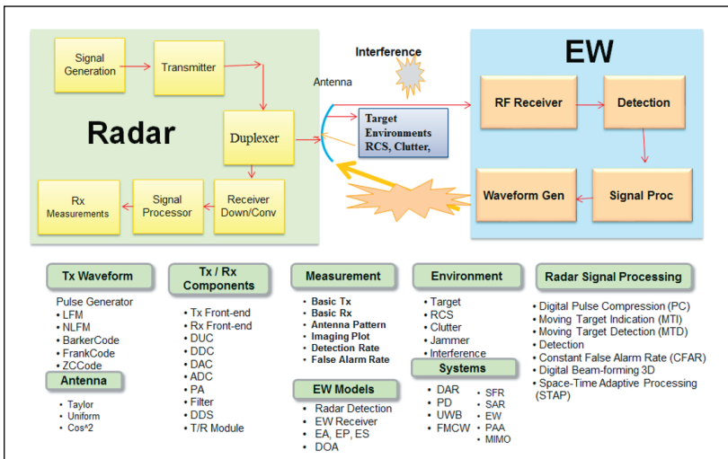
Рисунок 1. Платформа моделирования систем РЛС и РЭБ компании Keysight моделирует и имитирует системы РЛС и РЭБ на всех этапах разработки.
