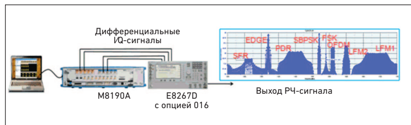
Рисунок 4. Здесь показан сигнал нескольких источников излучения, включающий составляющие сигналов различных РЛС и систем связи, сгенерированный с использованием платформы для тестирования систем РЛС и РЭБ на базе САПР SystemVue компании Keysight.
