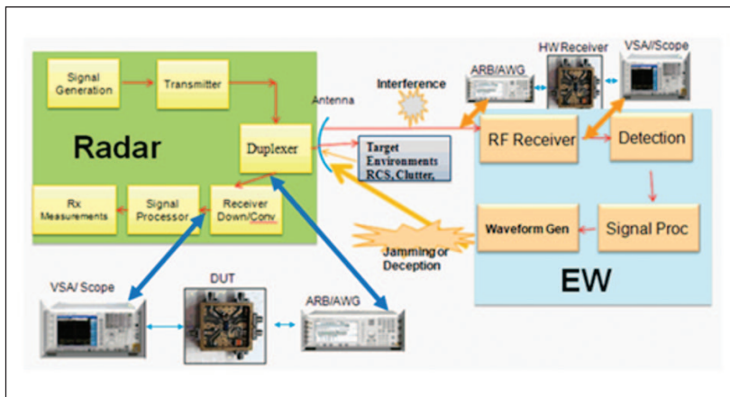
Рисунок 2. Платформа SystemVue для тестирования систем РЛС и РЭБ, которая может использоваться для тестирования и проверки аппаратных средств. На этой схеме показано, как сигнал, передаваемый РЛС, с помехой, имитируемой SystemVue, загружаются в генератор сигналов произвольной формы для тестирования аппаратных средств РЧ-приёмника системы РЭБ.
