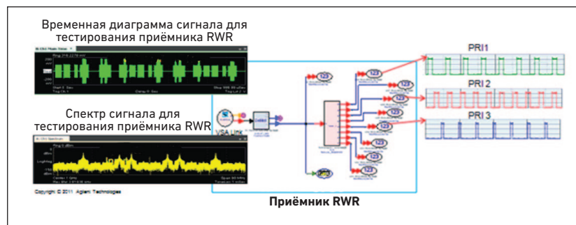
Рисунок 5. Этот шаблон платформы для испытания RWR использует метод распознавания полос частот (Frequency Bands Recognition). RWR базируется на обработке сигналов с частотным разделением каналов, обеспечивая восемь входов, для каждого из которых можно установить отличающийся диапазон частот.
