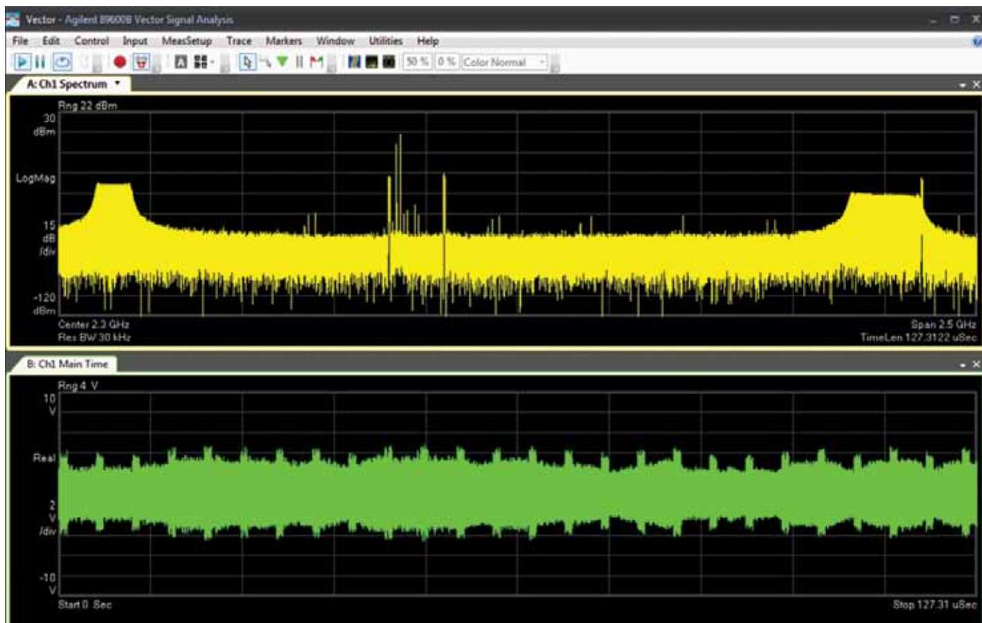
Рис. 6. Результаты измерений сигнала нескольких ИПИ, отображаемые на экране осциллографа DSA 91304A с ПО VSA.
