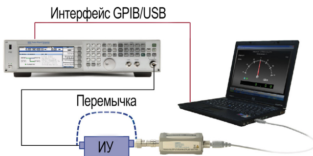
Рисунок 2 - Метод измерения с поствыравниванием по уровню является менее затратным при более высокой точности
