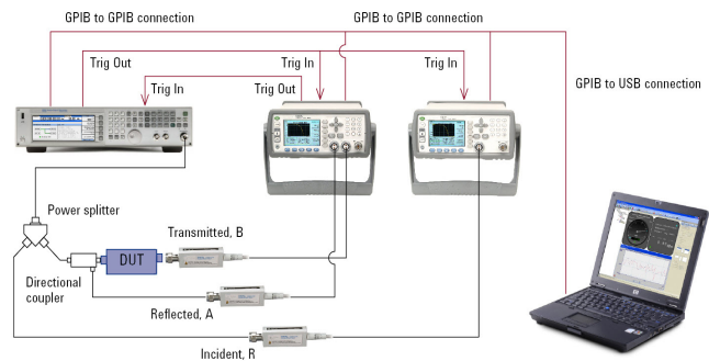
Рисунок 7 - Конфигурация установки с оптимизацией скорости измерения позволяет достичь 15 мс на отсчёт
