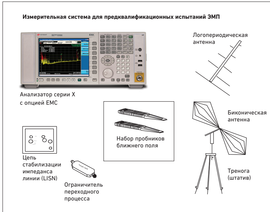
Рисунок 3. Компоненты системы для предварительной оценки уровня помех
