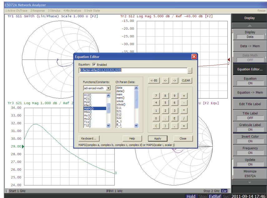
Рис. 2. Вычисление К-фактора с использованием редактора уравнений.
