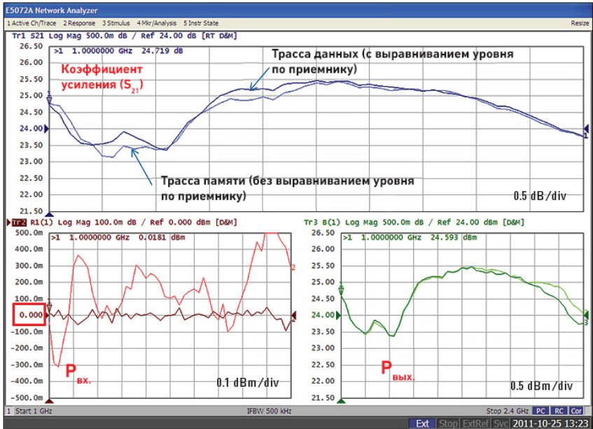
Рис. 28. Выравнивание уровня по приемнику позволяет повысить точность импульсных измерений усилителя в нелинейной области.
