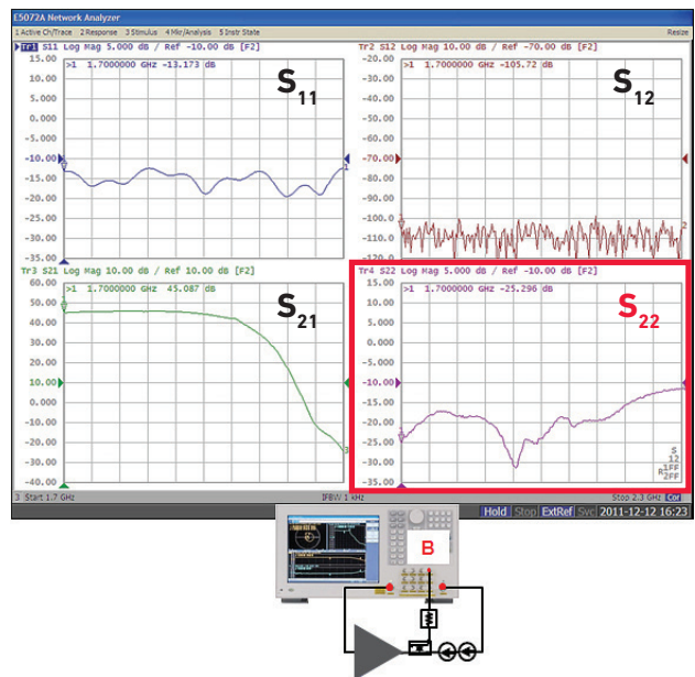
Рис. 5. Результат измерения усилителя мощности с использованием схемы измерений с прямым доступом к приемнику.
