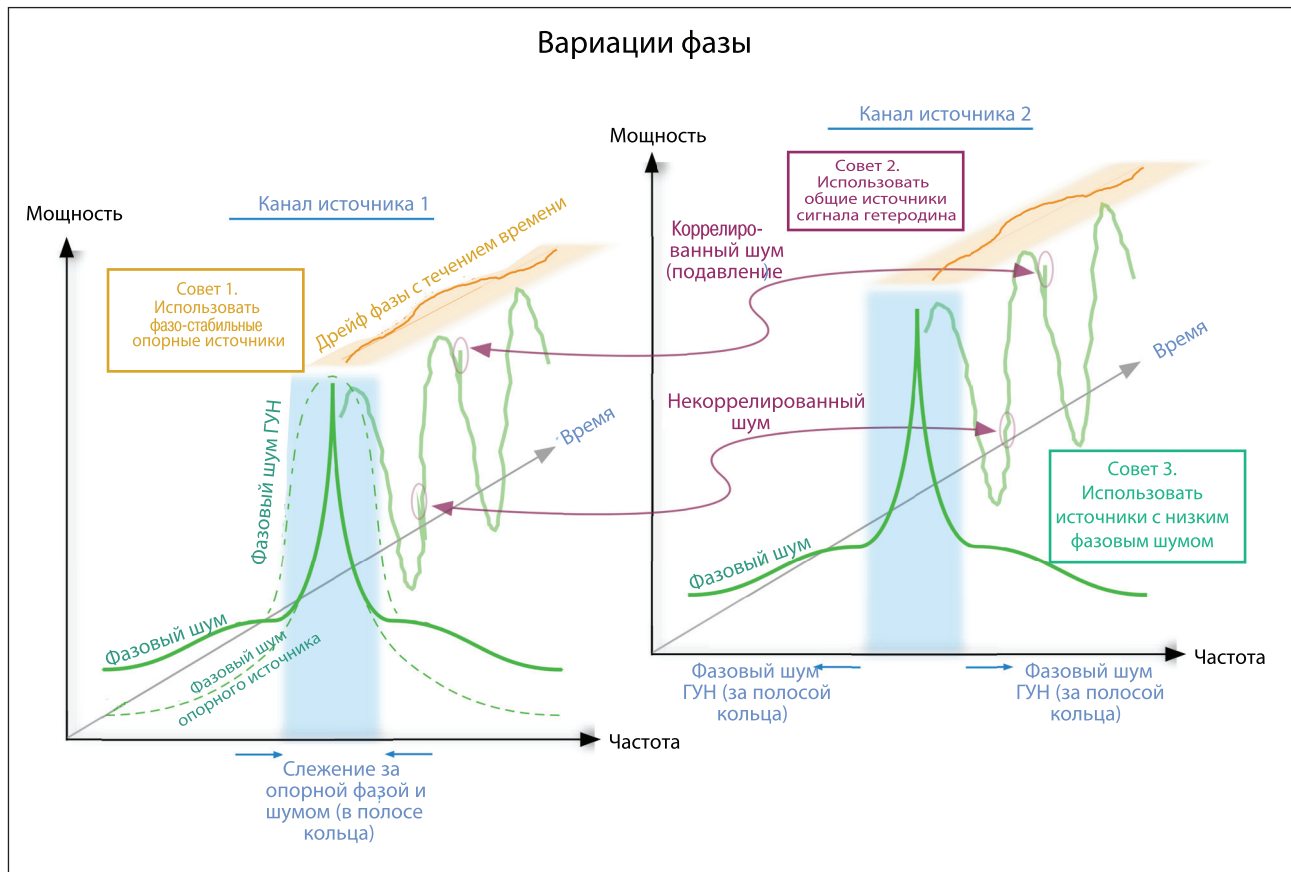
Рисунок 5. Фазовые вариации между источниками, синхронизированными общим опорным генератором в пределах полос пропускания их колец ФАП. Характеристики улучшаются при использовании высококачественного опорного источника и синхронизируемых приборов с низким уровнем фазового шума или при использовании для синхронизации более высокочастотного опорного источника или гетеродинов (LO).
