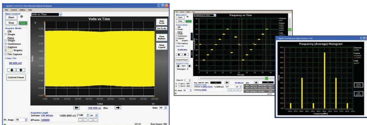
Рисунок 6 - Изображение слева показывает осциллограмму ВЧ сигнала со скачкообразной перестройкой частоты. Изображение в центре представляет скачкообразные частоты и продолжительность генерации каждой частоты. Изображение справа, гистограмма, показывает число импульсов для каждой частоты.
