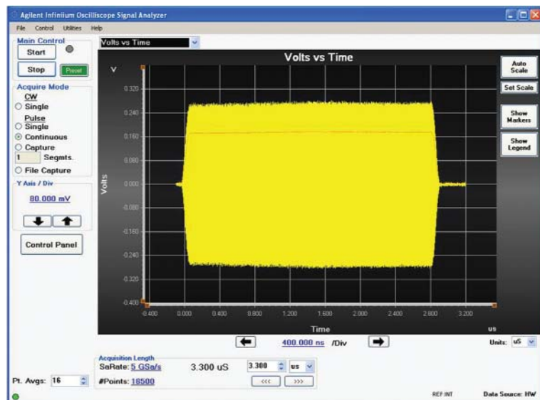
Рисунок 1- Возможности программы OSA позволяют выполнять измерения импульсных и непрерывных ВЧ сигналов, а также анализ сигналов в модуляционной области. В режиме работы с импульсными и непрерывными сигналами данные измерений отображаются в единицах напряжения (вольт) в зависимости от времени, подобно типичному осциллографическому отображению. Доступны также и другие режимы измерения.
